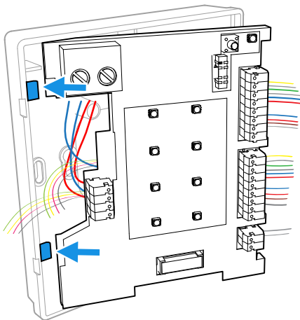
Abb. 9: Leiterplatte in das Gehäuseunterteil einsetzen
