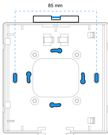
Abb. 4: Äußere Befestigungspunkte anzeichnen
