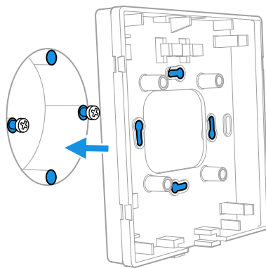
Abb. 5: Befestigung auf einer Standard-Installationsdose
