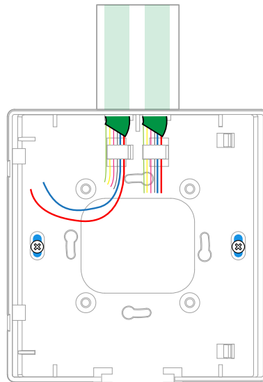
Abb. 8: Leitungen bei aP-Montage
