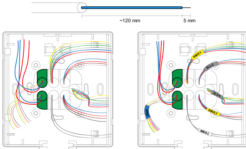
Abb. 6: Leitungsführung bei Montage auf Standard-Installationsdose
