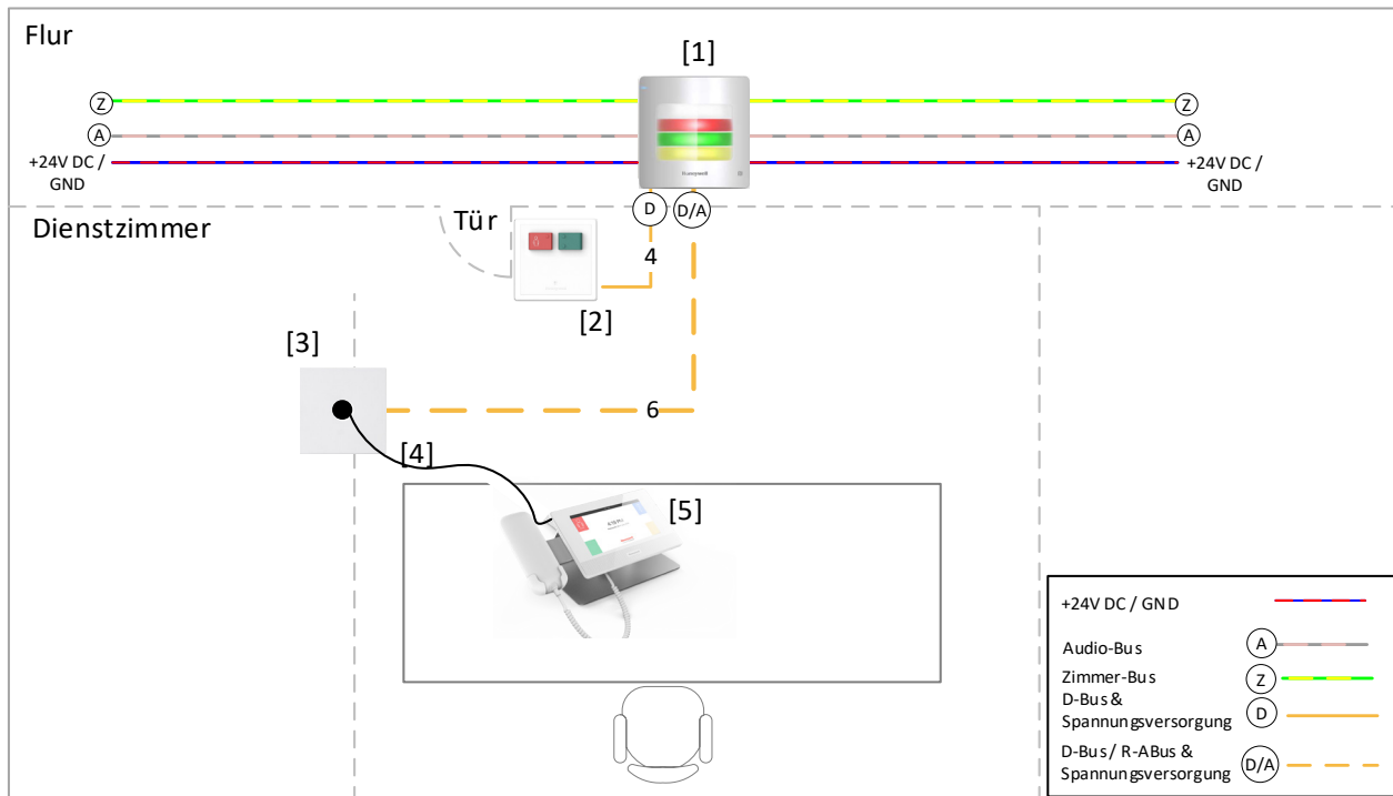
Abb. 15: Schematische Anschaltung
