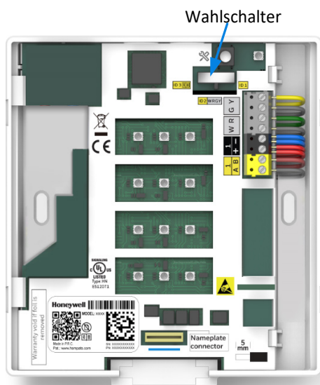
Abb. 16: Platine SCL, Wahlschalter werkseitig in Position ID1
