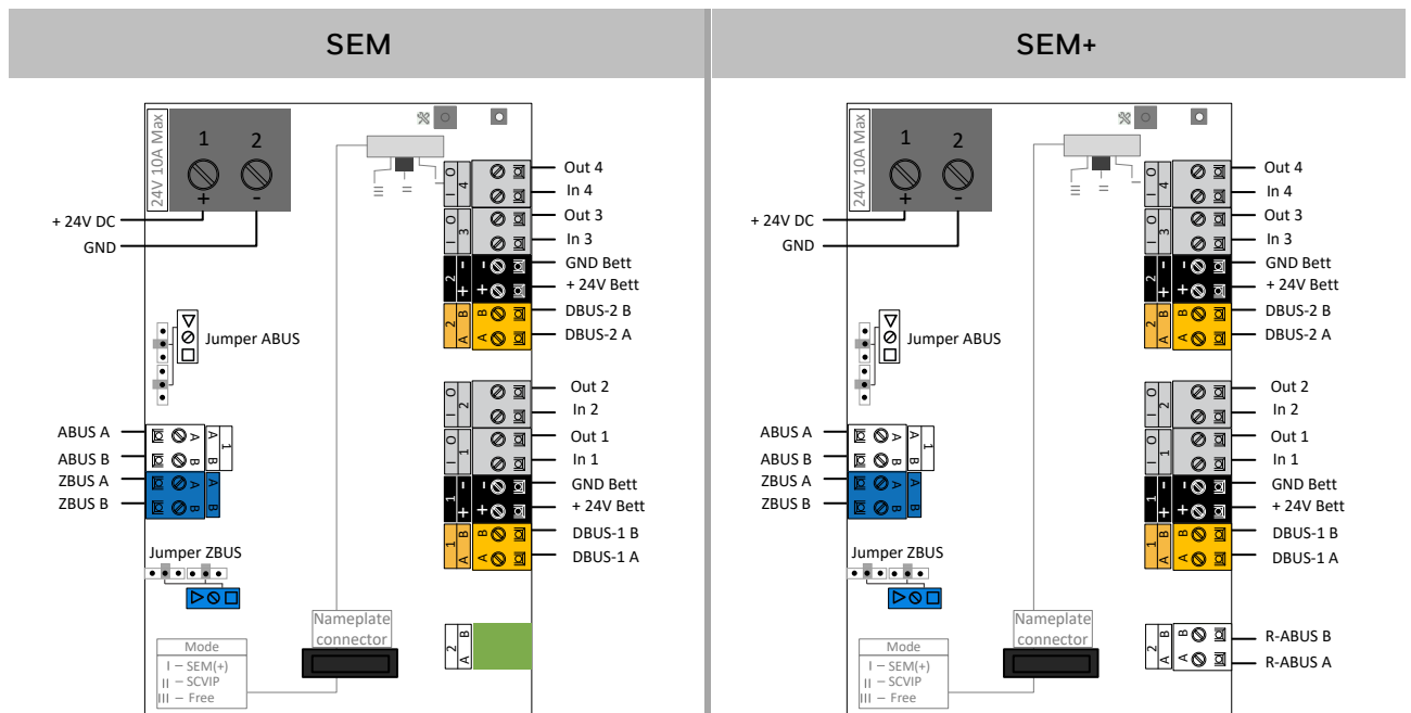
Abb. 13: Anschlussklemmen SEM
