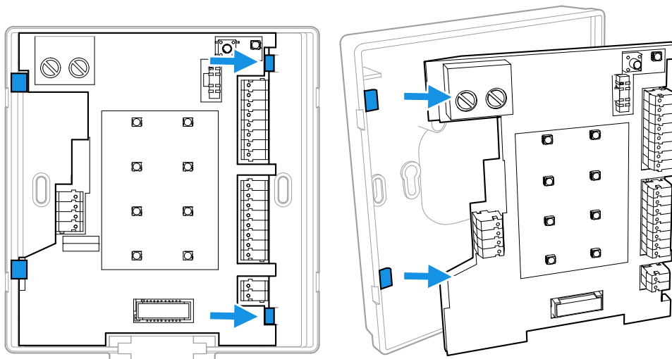
Abb. 2: Leiterplatte aus dem Gehäuseunterteil entnehmen
