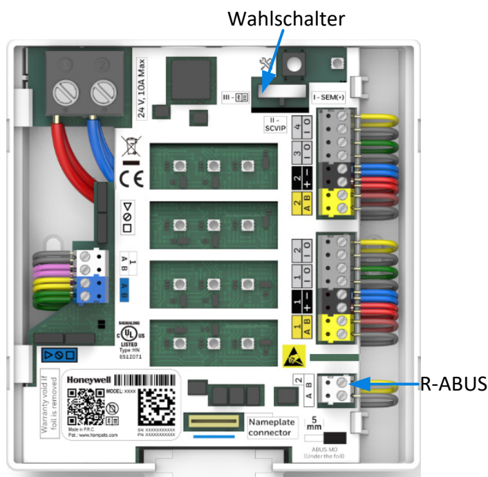
Abb. 12: Platine SEM / SEM+ Wahlschalter ab Werk in Position I-SEM(+)
