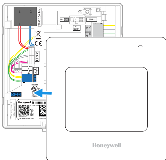
Abb. 11: Abdeckung mit Leuchtschale aufsetzen
