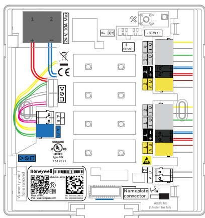
Abb. 10: Anschlussklemmen aufstecken und Leitungen führen
