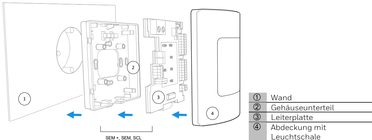
Abb. 3: Montage auf der Wand
